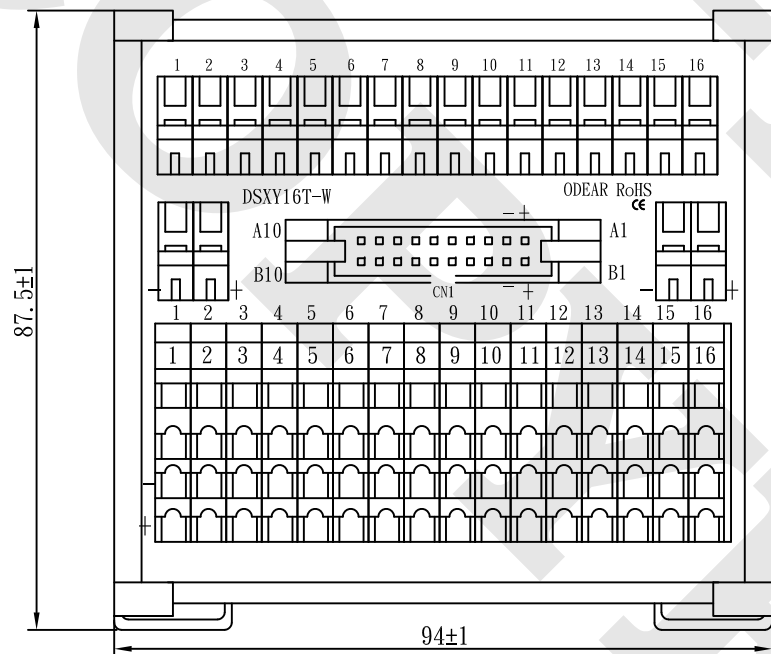
IDC腳位圖：
