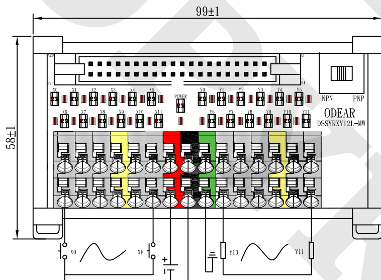
此圖為外部配線圖
