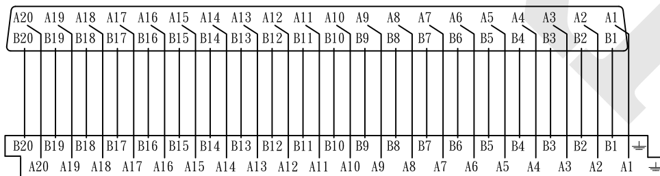
IDC腳位圖：
