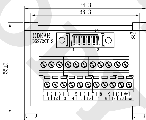
腳位圖：
