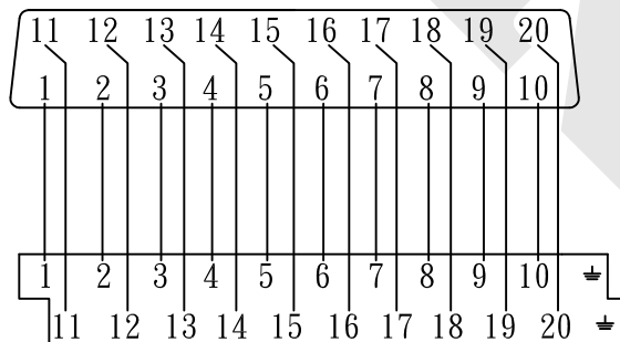
腳位圖：
