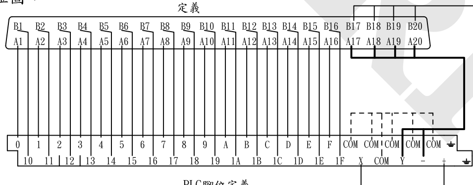
PLC腳位定義
