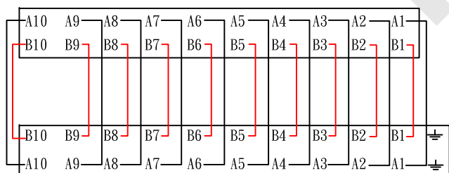
腳位圖:
