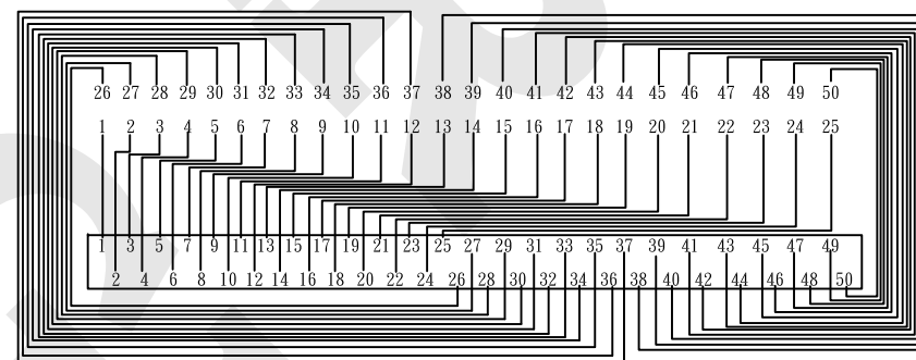
腳位圖:
