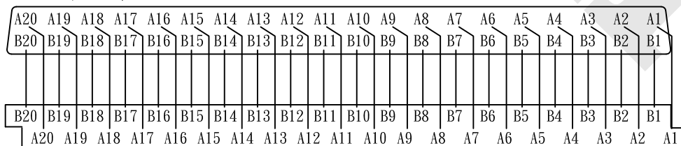
IDC腳位圖：
