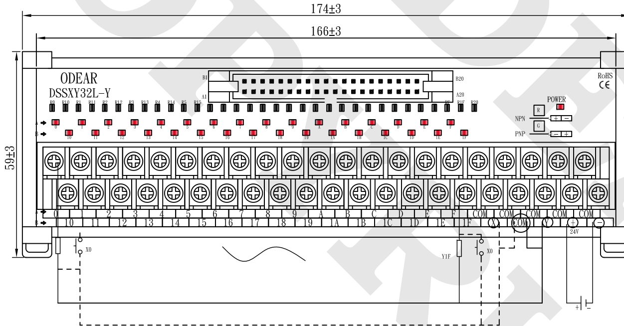
此圖為 NPN 之外部配線圖
