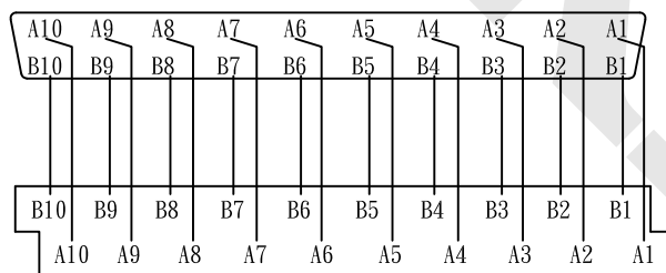
腳位圖1:
