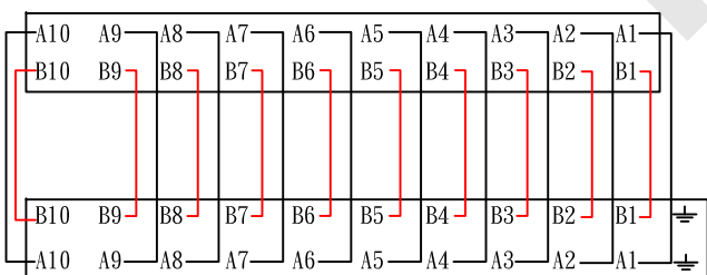
腳位圖:
