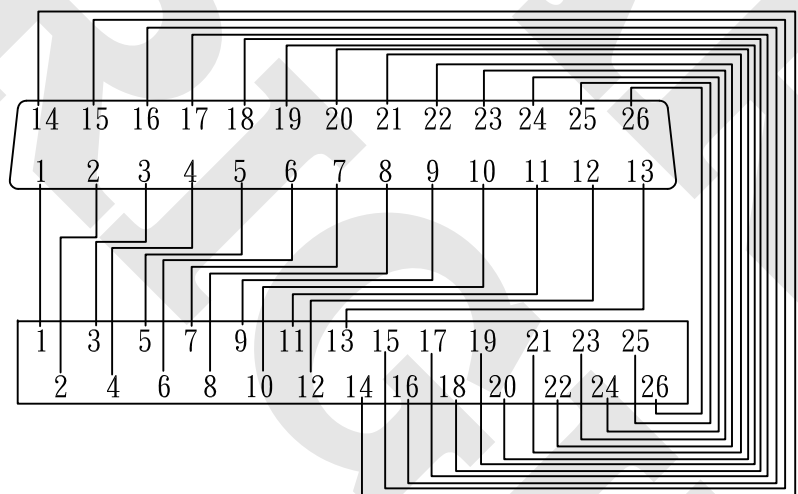
腳位圖:
